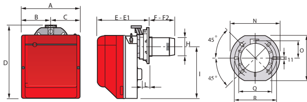
RS 5 - RS 5D BRÜLÖRLERDE GENEL ÖLÇÜLER mm
