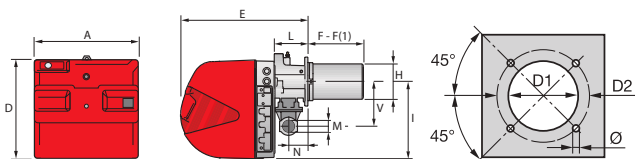
RS 34/1 BRÜLÖRLERDE GENEL ÖLÇÜLER mm
